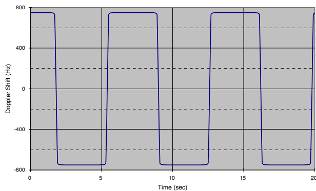
Figure B.3-1: Doppler shift trajectory
