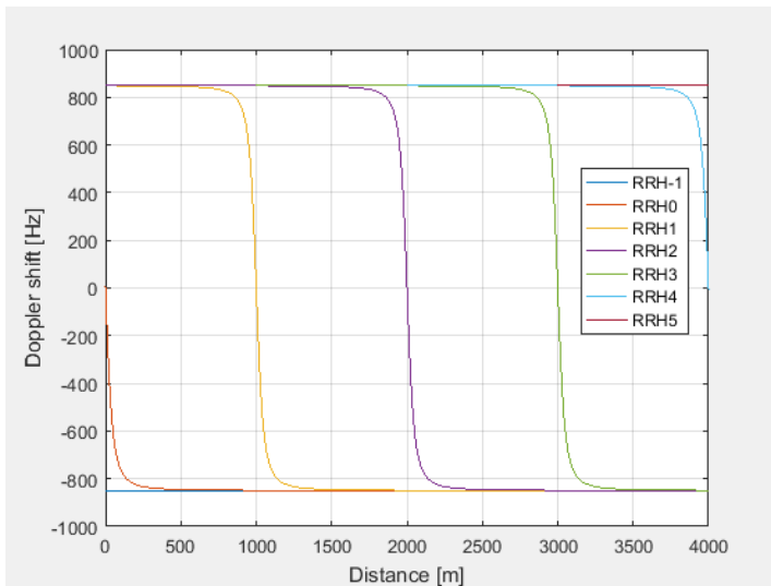
Figure B.3A-3 Doppler shifts trajectories
