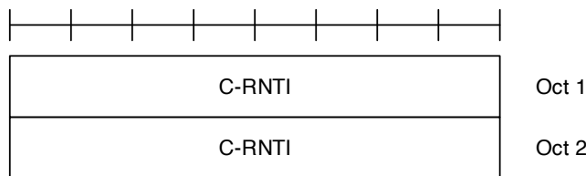
Figure 6.1.3.2-1: C-RNTI MAC CE
